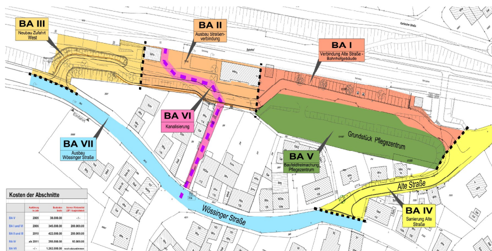
Darstellung der 7 Bauabschnitte
